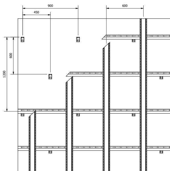
Fasadevekt maks. 430 kg/m   (sikksakkmontering)
