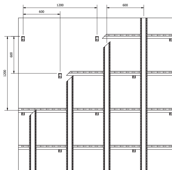
Fasadevekt maks. 70 kg/m  
