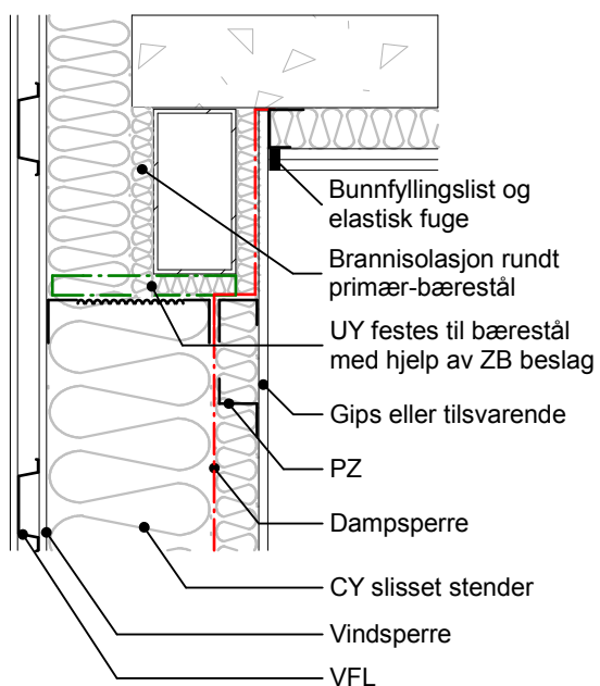
Mot stålbering
