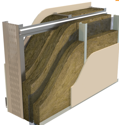
Tosidig staget
